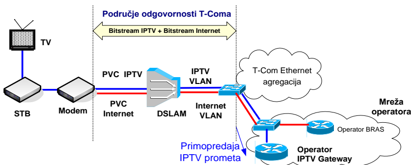
Slika 2627. Veleprodajni širokopojsni pristup za pružanje IPTV usluge preko ADSL/VDSL pristupa na DSLAM razini
