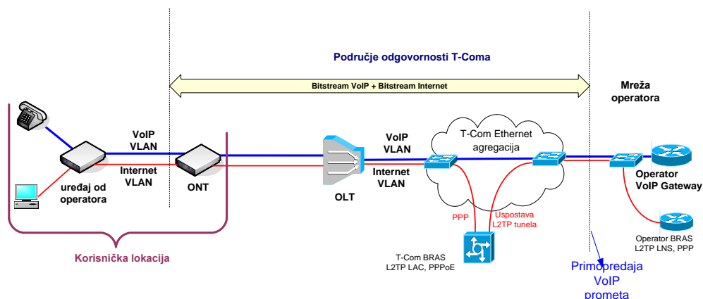
Slika 4213. Realizacija posebnog virtualnog kanala za VoIP uslugu preko FTTH pristupa (GPON)
