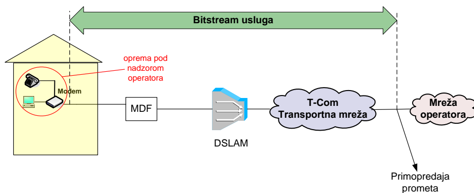
Slika 910. Koncept posebnog virtualnog kanala za VoIP uslugu u slučaju kada Krajnji korisnik ostvaruje Osnovni pristup mreži putem usluge T-Coma
