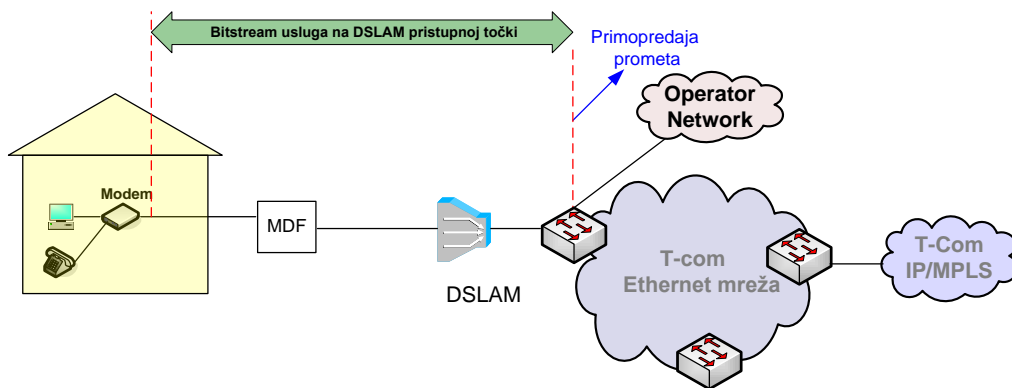
| Slika 67. Veleprodajni širokopolasni pristup za pružanje Internet usluge na DSLAM razini u slučaju kada Krajnji korisnik ostvaruje Osnovni pristup mreži putem usluge T-Coma
