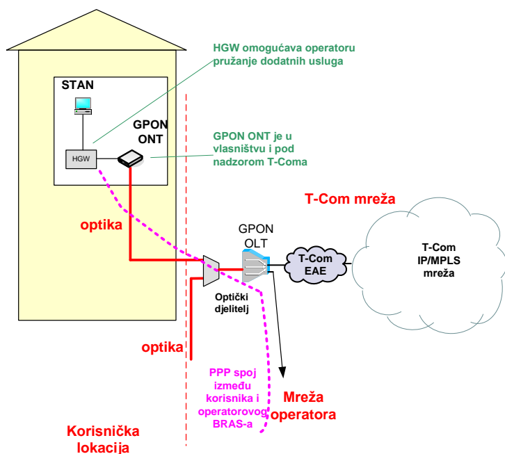
Slika 56. Način realizacije usluge veleprodajnog širokopojasnog pristupa za Internet uslugu na temelju FTTH tehnologije rješenja na OLT razini
