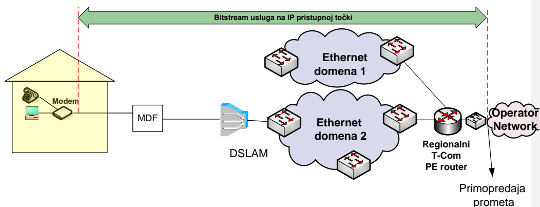
Slika 4617. Veleprodajni širokopolasni pristup za pružanje VoIP usluge na IP razini u slučaju kada Krajnji korisnik ostvaruje Osnovni pristup mreži putem usluge Operatora korisnika
