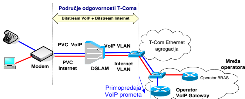
Slika 4819. Veleprodajni širokopolasni pristup za pružanje VoIP usluge preko ADSL/VDSL pristupa na DSLAM razini
