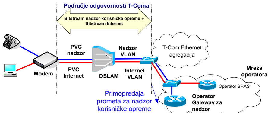
Slika 2829. Veleprodajni širokopojasni pristup za pružanje usluge nadzora korisničke opreme preko ADSL/VDSL pristupa na DSLAM razini
