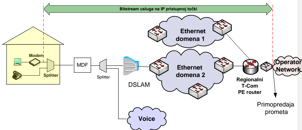
Slika 1516. Veleprodajni širokopolasni pristup za pružanje VoIP usluge na IP razini u slučaju kada Krajnji korisnik ostvaruje Osnovni pristup mreži putem usluge T-Coma
