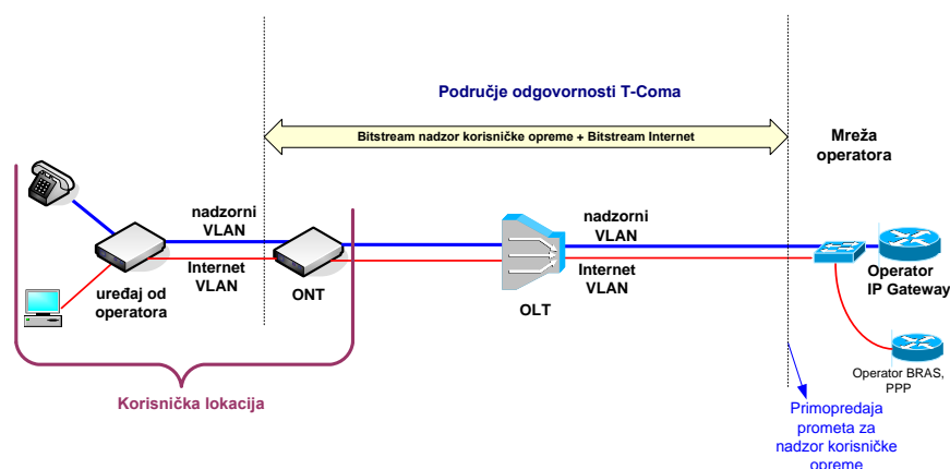
Slika 2728. Veleprodajni širokopojasni pristup za pružanje usluge nadzora korisničke opreme preko FTTH pristupa (GPON) na OLT razini
