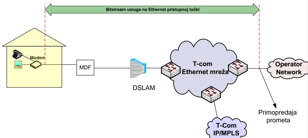
Slika 1415. Veleprodajni širokopolasni pristup za pružanje VoIP usluge na Ethernet razini u slučaju kada Krajnji korisnik ostvaruje Osnovni pristup mreži putem usluge Operatora korisnika
