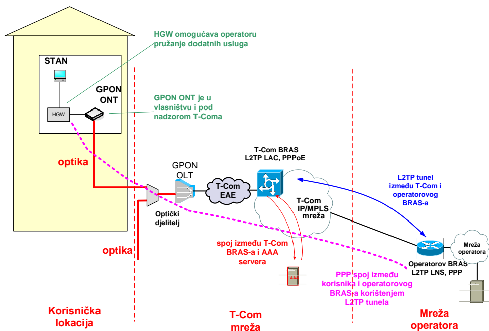
Slika 2. Način realizacije usluge veleprodajnog širokopojsnog pristupa za Internet uslugu na temelju FTTH tehnologije rješenja na IP razini
