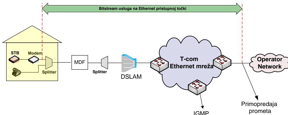
Slika 2324. IPTV usluga na Ethernet razini putem ADSL/VDSL tehnologije u slučaju kada Krajnji korisnik ostvaruje Osnovni pristup mreži putem usluge T-Coma
