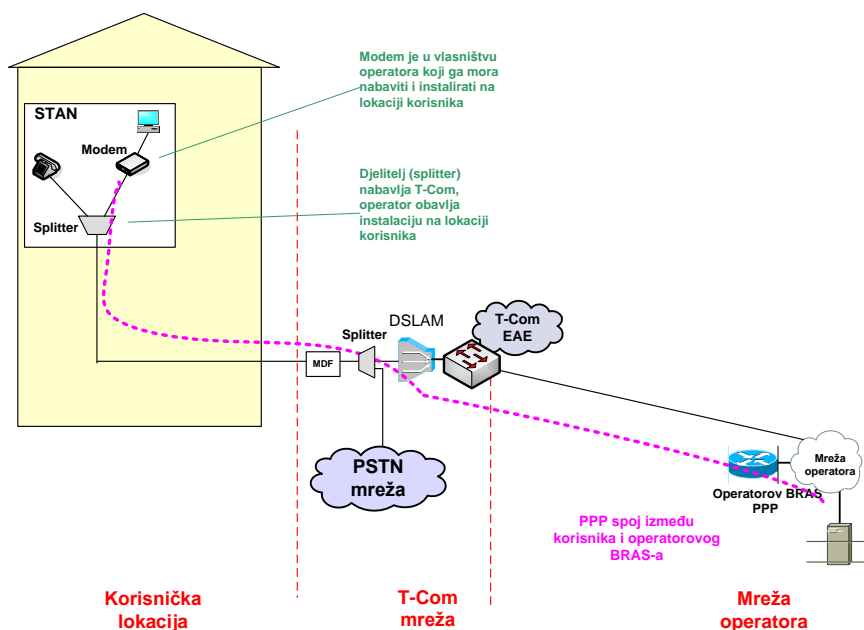
Slika 89. Način realizacije Veleprodajnog širokopojasnog pristupa za pružanje Internet usluge na DSLAM razini
