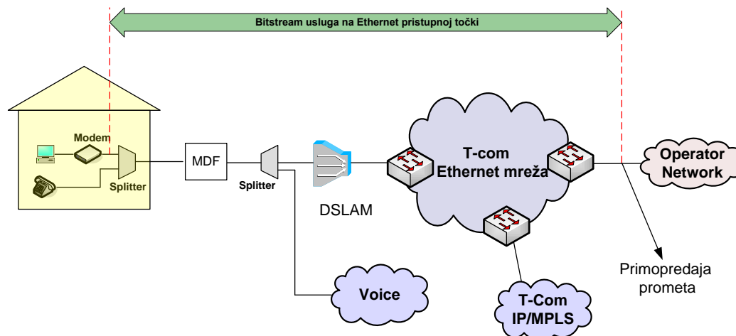
Slika 4314. Veleprodajni širokopolasni pristup za pružanje VoIP usluge na Ethernet razini u slučaju kada Krajnji korisnik ostvaruje Osnovni pristup mreži putem usluge T-Coma
