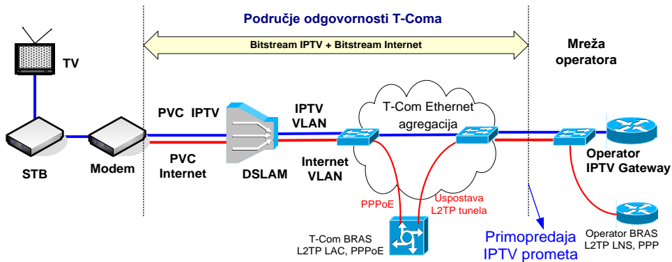
Slika 2122. Realizacija posebnog virtualnog kanala za IPTV uslugu preko ADSL/VDSL pristupa (kod VDSL pristupa između modema i DSLAM-a koristi se odgovarajući VLAN)
