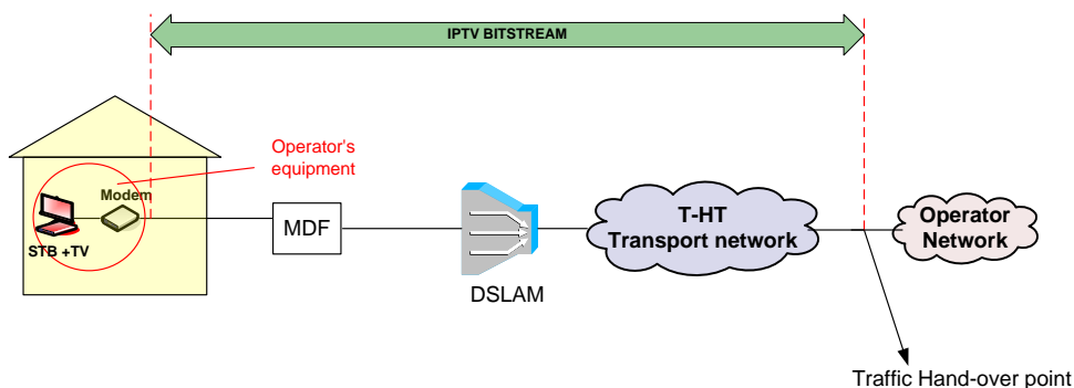
Slika 2021. Koncept posebnog virtualnog kanala za IPTV uslugu u slučaju kada Krajnji korisnik ostvaruje Osnovni pristup mreži putem usluge Operatora korisnika
