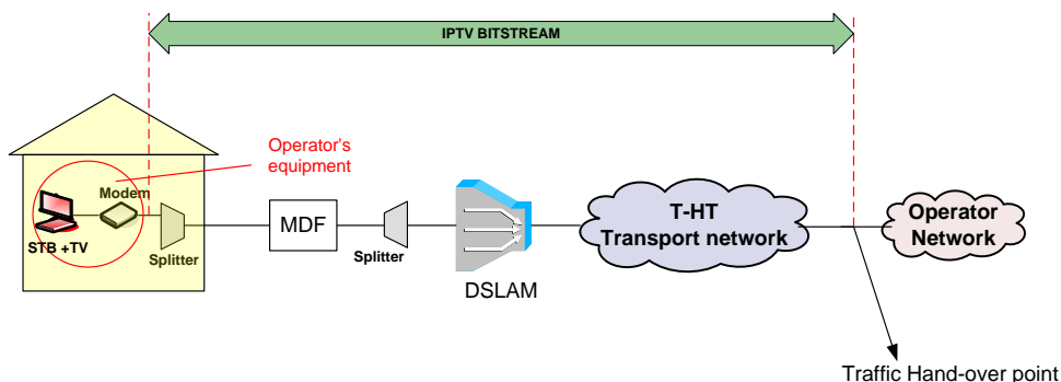
Slika 1920. Koncept posebnog virtualnog kanala za IPTV uslugu u slučaju kada Krajnji korisnik ostvaruje Osnovni pristup mreži putem usluge T-Coma
