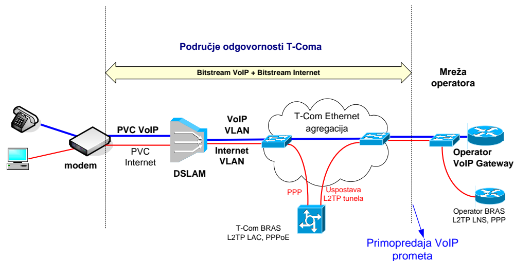
Slika 4.12. Realizacija posebnog virtualnog kanala za VoIP uslugu preko ADSL/VDSL pristupa (kod VDSL pristupa između modema i DSLAM-a koristi se odgovarajući VLAN)
