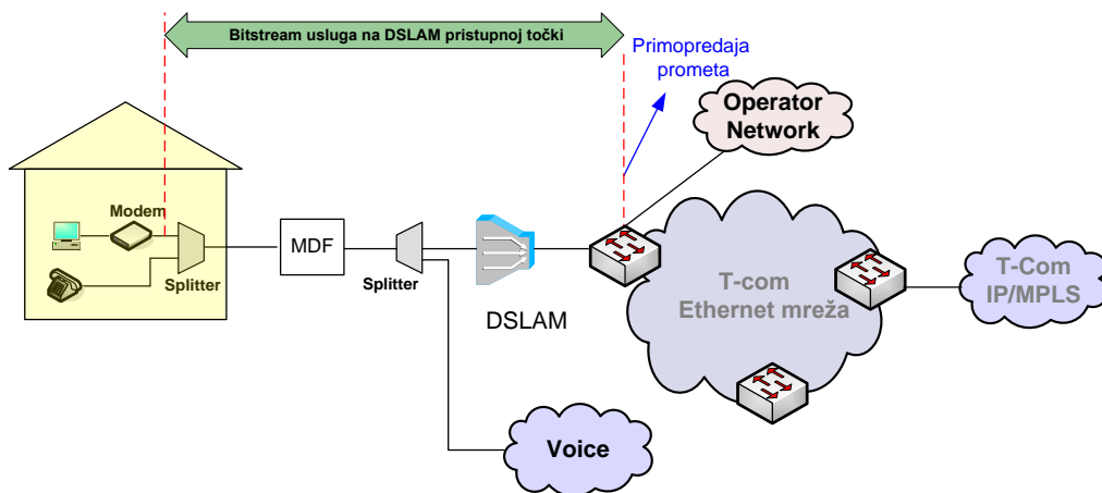
| Slika 67. Veleprodajni širokopolasni pristup za pružanje Internet usluge na DSLAM razini u slučaju kada Krajnji korisnik ostvaruje Osnovni pristup mreži putem usluge T-Coma
