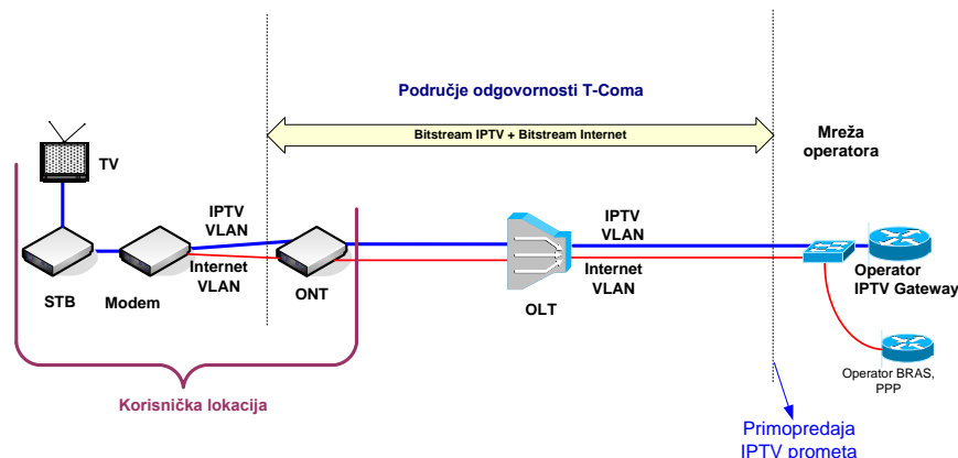
Slika 2526. Veleprodajni širokopojsni pristup za pružanje IPTV usluge preko FTTH pristupa (GPON) na OLT razini
