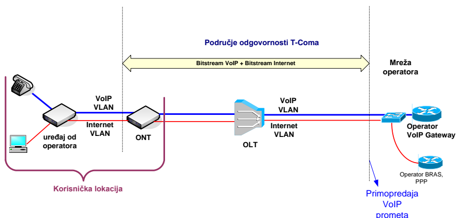
Slika 4718. Veleprodajni širokopolasni pristup za pružanje VoIP usluge preko FTTH pristupa (GPON) na OLT razini
