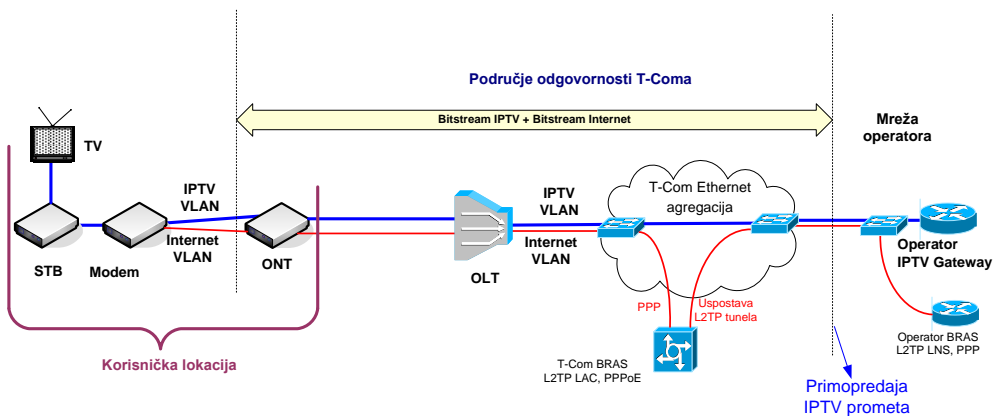
Slika 2223. Realizacija posebnog virtualnog kanala za IPTV uslugu preko FTTH pristupa (GPON)
